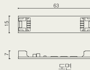
서브컨트롤러 KCL-SC-01
